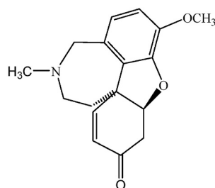
Narwedine
