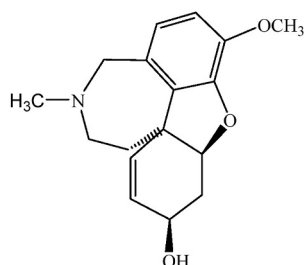
Galantamine
